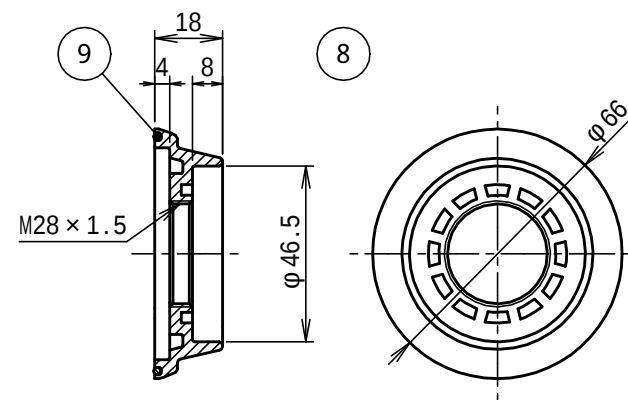
座付化粧リング
