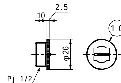
継手キャップ
